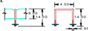
DETALLE DE AGARRADERA
