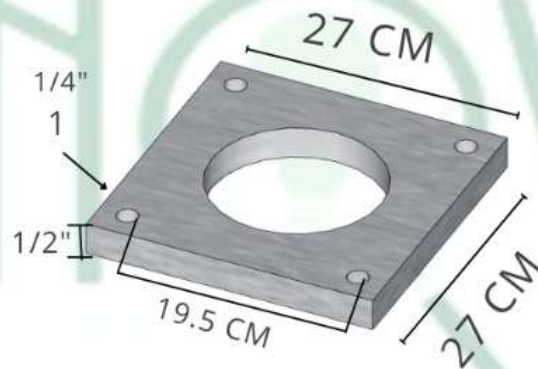
PLACA BASE DE 0.27 X 0.27 M
